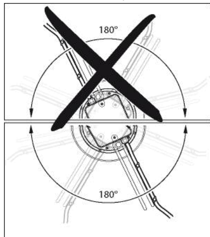
Illustr. 3: Pose des câbles pour ventilateurs montés debout.
