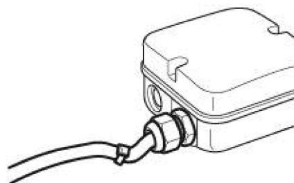
Illustr. 1: Ventilateur monté couché, pose du câble avec boucle de détente de contrainte.
