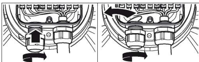
Illustr. 4: Percement presse-câble fileté
